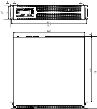
Рисунок 3а. Габаритные размеры и компоненты ИБП Штиль STR500SL и STR500SL-18 (горизонтальная установка в стойку)
