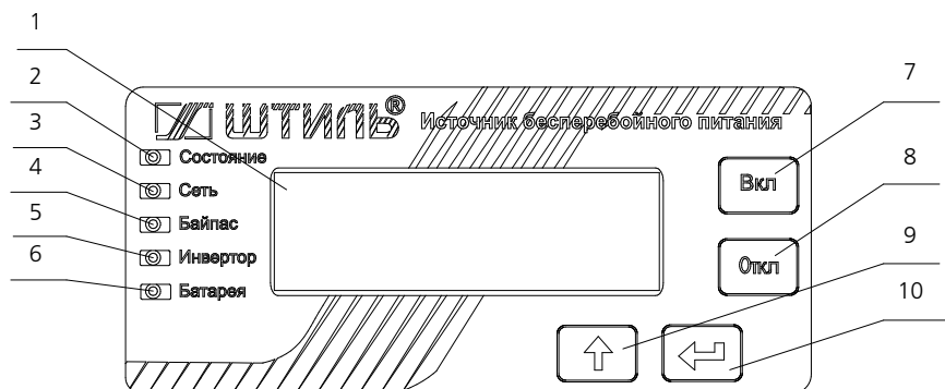
Рисунок 7а. Панель управления и индикации Штиль STR500SL и STR500SL-18
