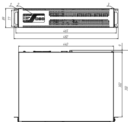
Рисунок 2а. Габаритные размеры и компоненты ИБП Штиль STR300SL и STR300SL-27 (горизонтальная установка в стойку)
